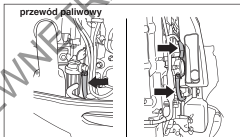
przewód paliwowy
